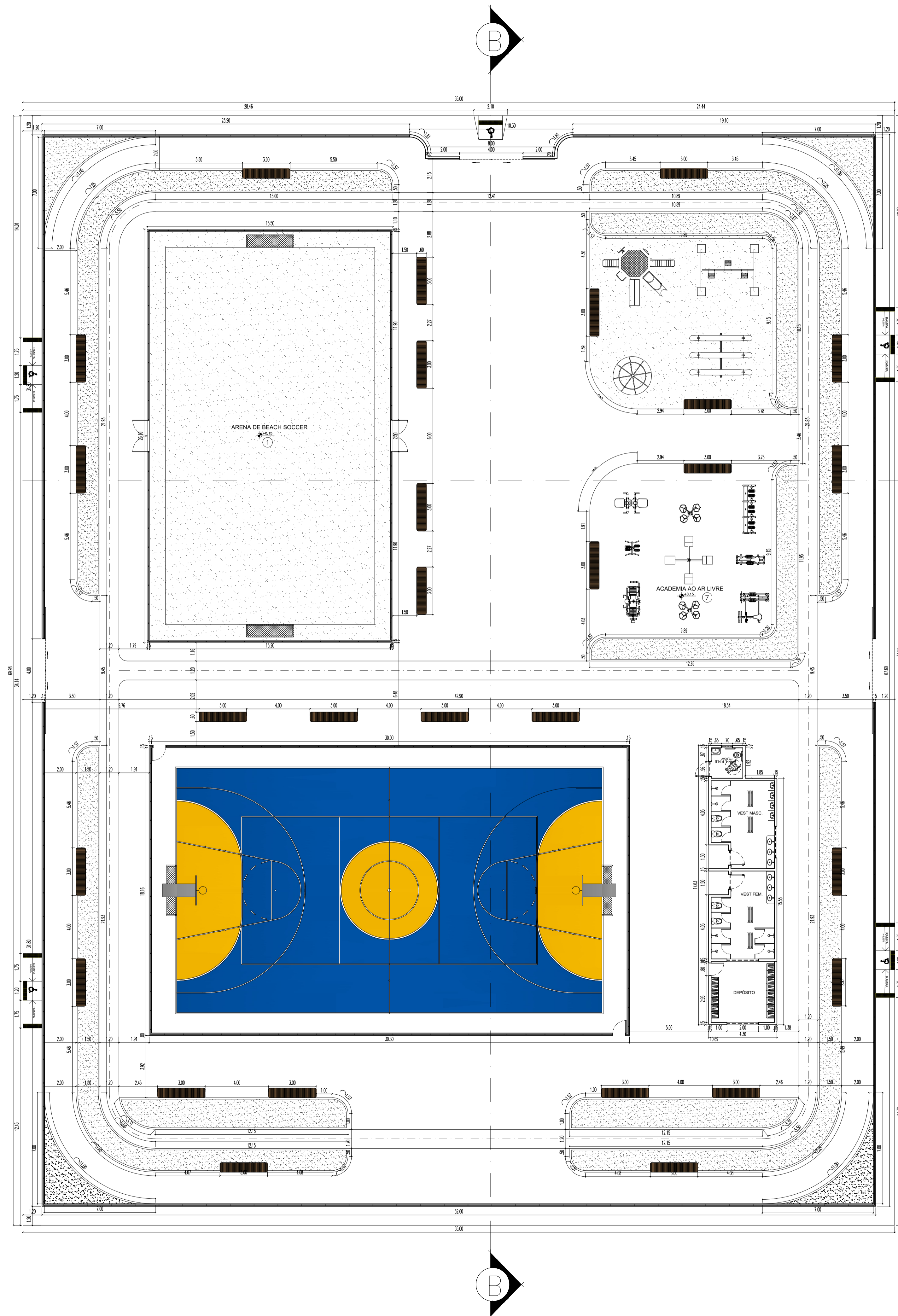
PLANTA BAIXA ESC. 1:150
